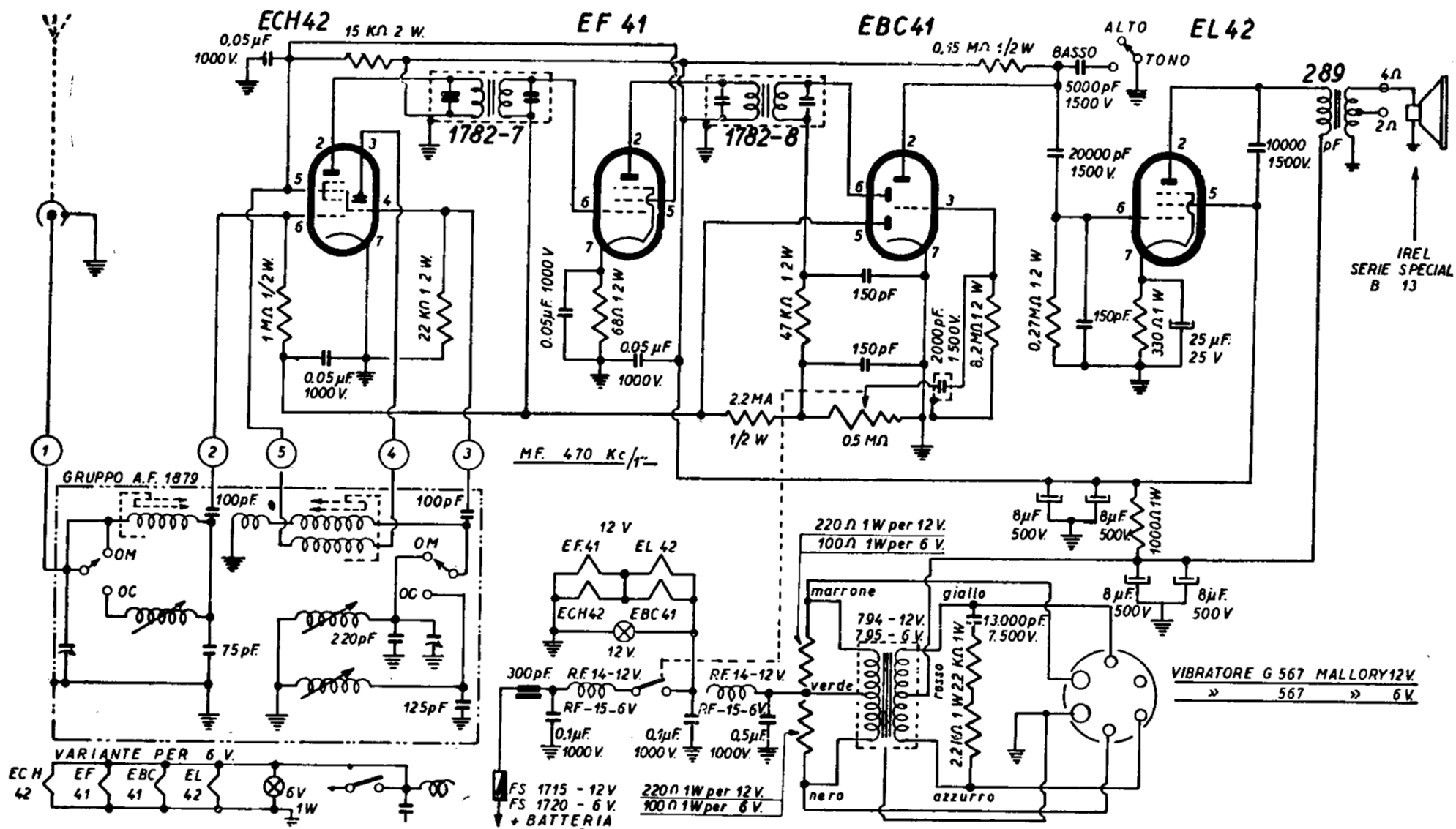
GALLO-CONDOR - AUTORADIO mod. « CONDORINO ». Una gamma onde medie ed una gamma onde corte. Sintonia a permeabilità variabile. Media frequenza 470 kc/s. Alimentazione a 12 o 6 volt, con sostituzione del vibratore, del fusibile, delle resistenze sul primario del trasformatore, ed effettuando la commutazione dei filamenti.
